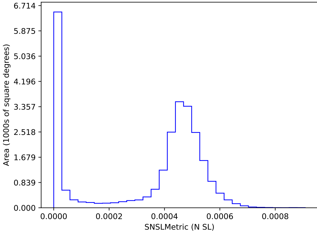
start_date_do270v3.4_10yrs : SNSLMetric
