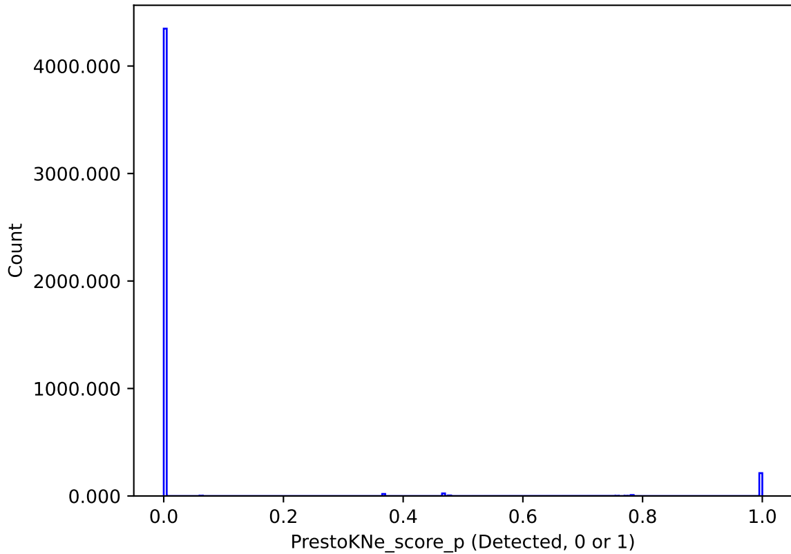
start_date_do270v3.4_10yrs : PrestoKNe_score_p
