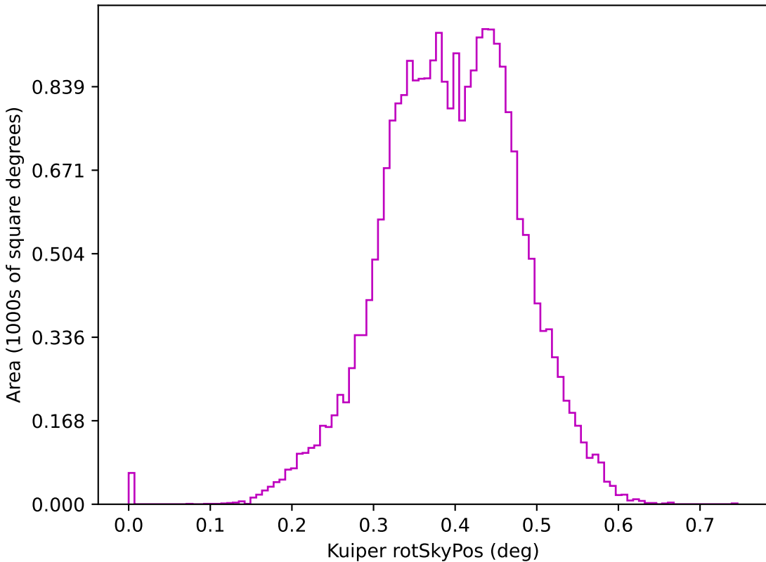
start_date_do270v3.4_10yrs z: Kuiper rotSkyPos
