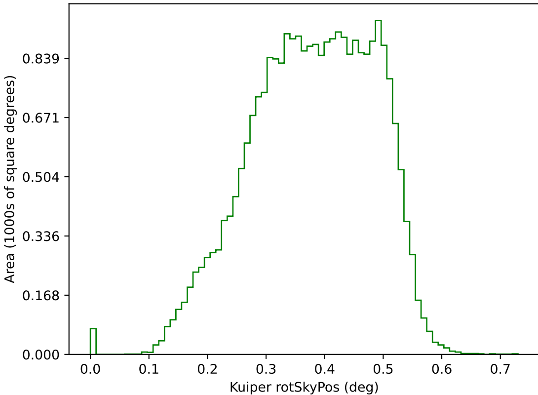
start_date_do270v3.4_10yrs g: Kuiper rotSkyPos
