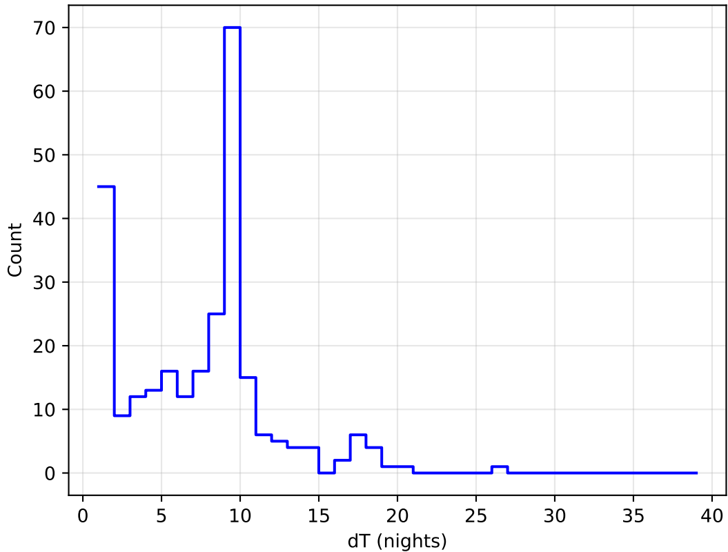
start_date_do270v3.4_10yrs all bands: DD:ELAISS1 Delta Nights Histogram
