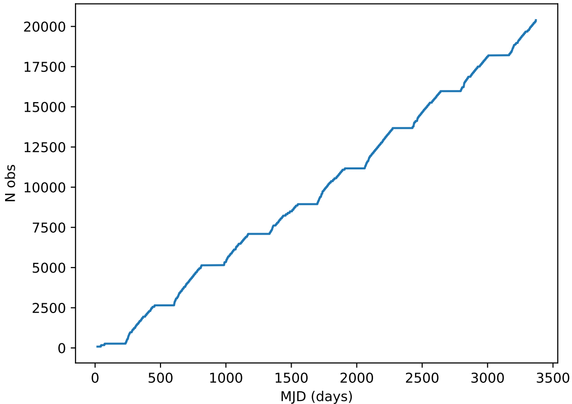
start_date_do180v3.4_10yrs all bands: DD:ELAISS1 Cumulative NVisits
