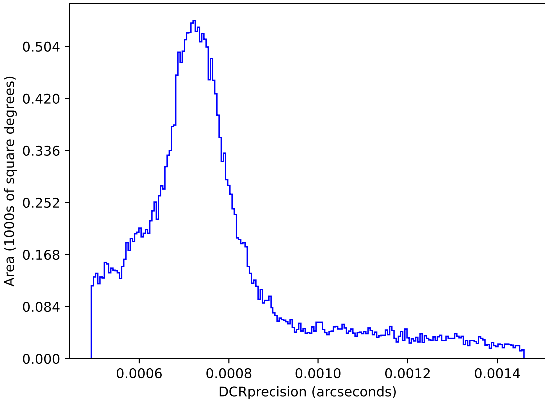
start_date_do0v3.4_10yrs : DCRprecision
