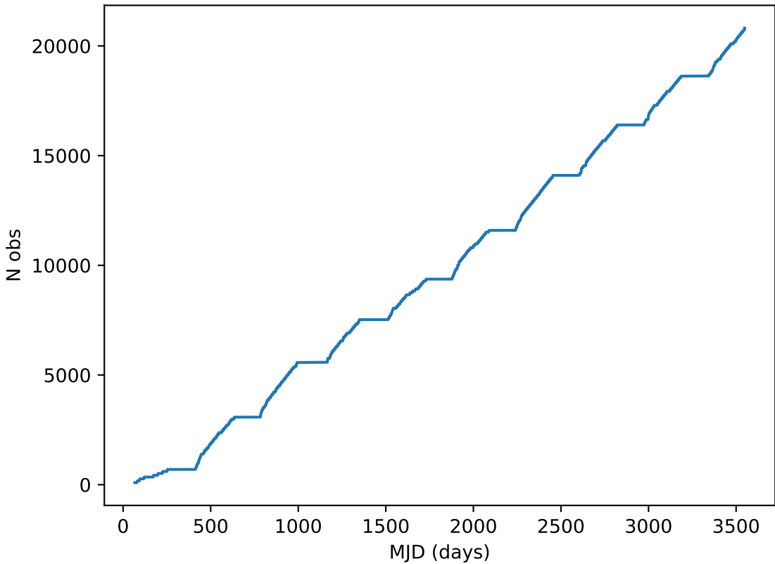
start_date_do0v3.4_10yrs all bands: DD:ELAISS1 Cumulative NVisits
