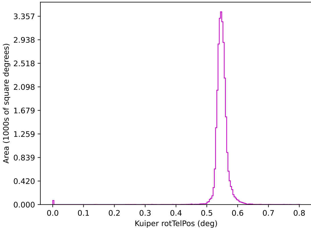
start_date_do-360v3.4_10yrs z: Kuiper rotTelPos
