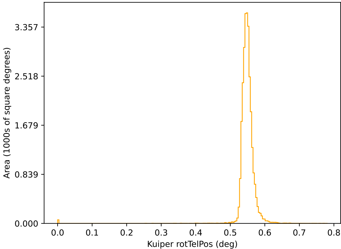
start_date_do-360v3.4_10yrs r: Kuiper rotTelPos
