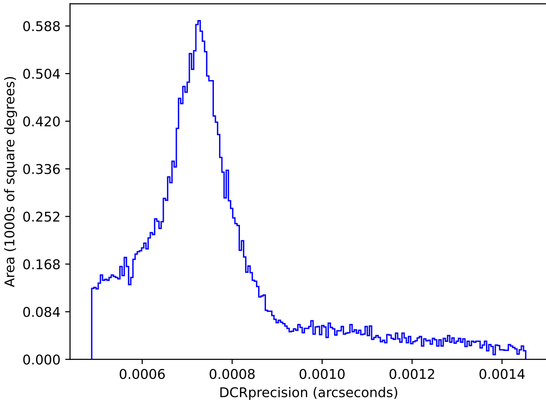
start_date_do-360v3.4_10yrs : DCRprecision
