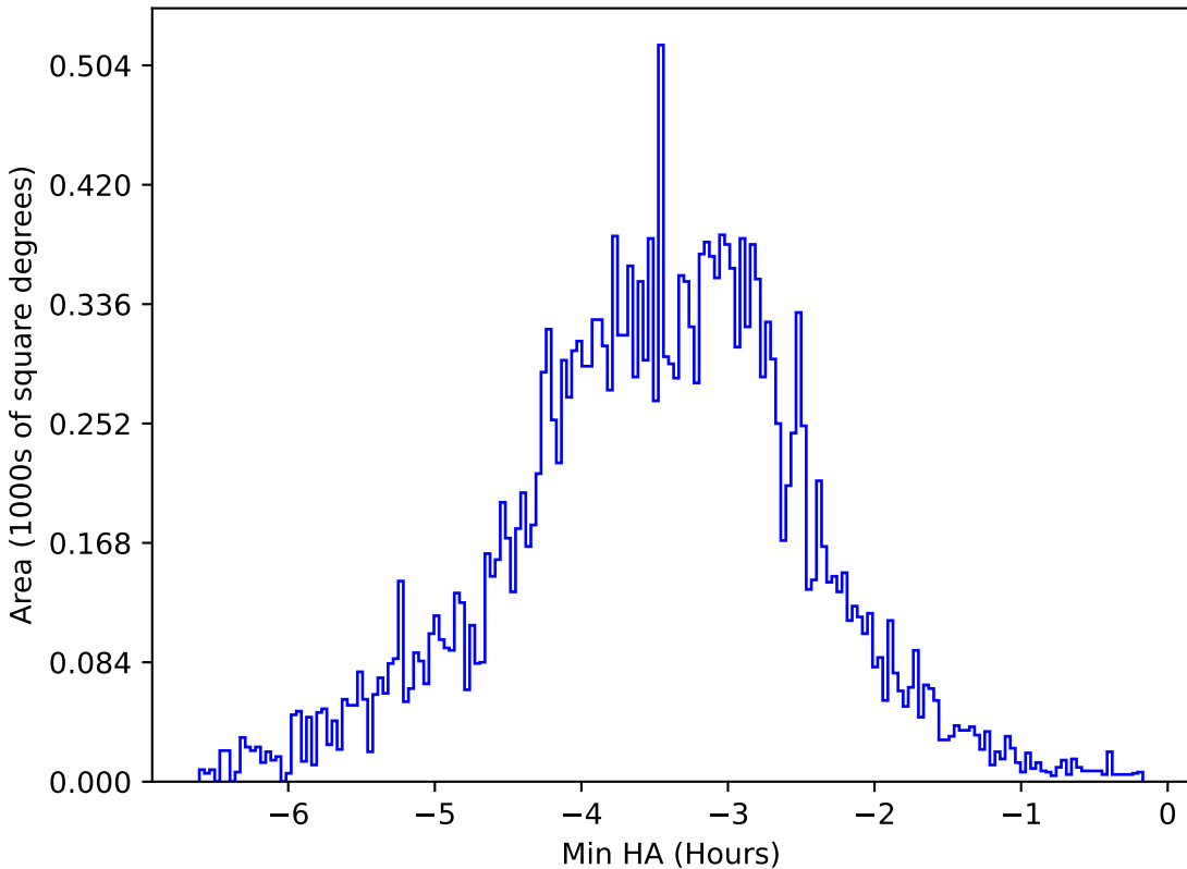
start_date_do-360v3.4_10yrs All sky y band: Min HA
