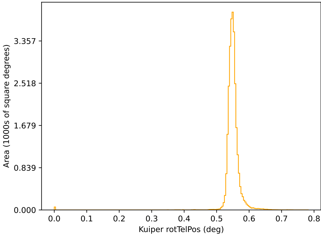
start_date_do-270v3.4_10yrs r: Kuiper rotTelPos
