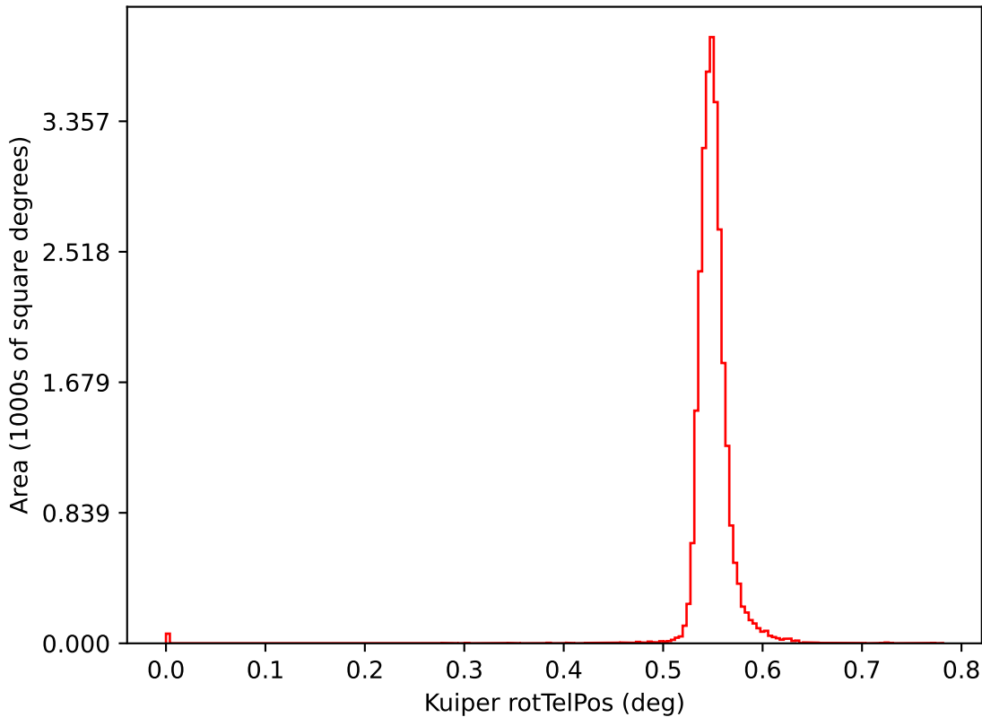
start_date_do-270v3.4_10yrs i: Kuiper rotTelPos
