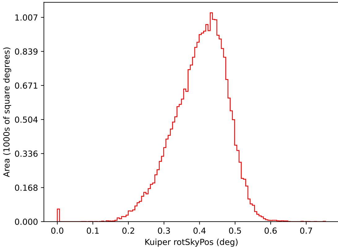
start_date_do-270v3.4_10yrs i: Kuiper rotSkyPos
