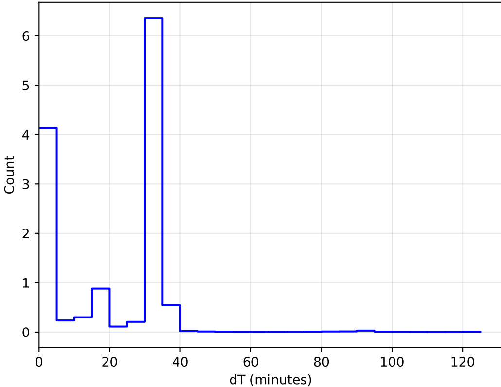
start_date_do-270v3.4_10yrs All sky: DeltaT Histogram
