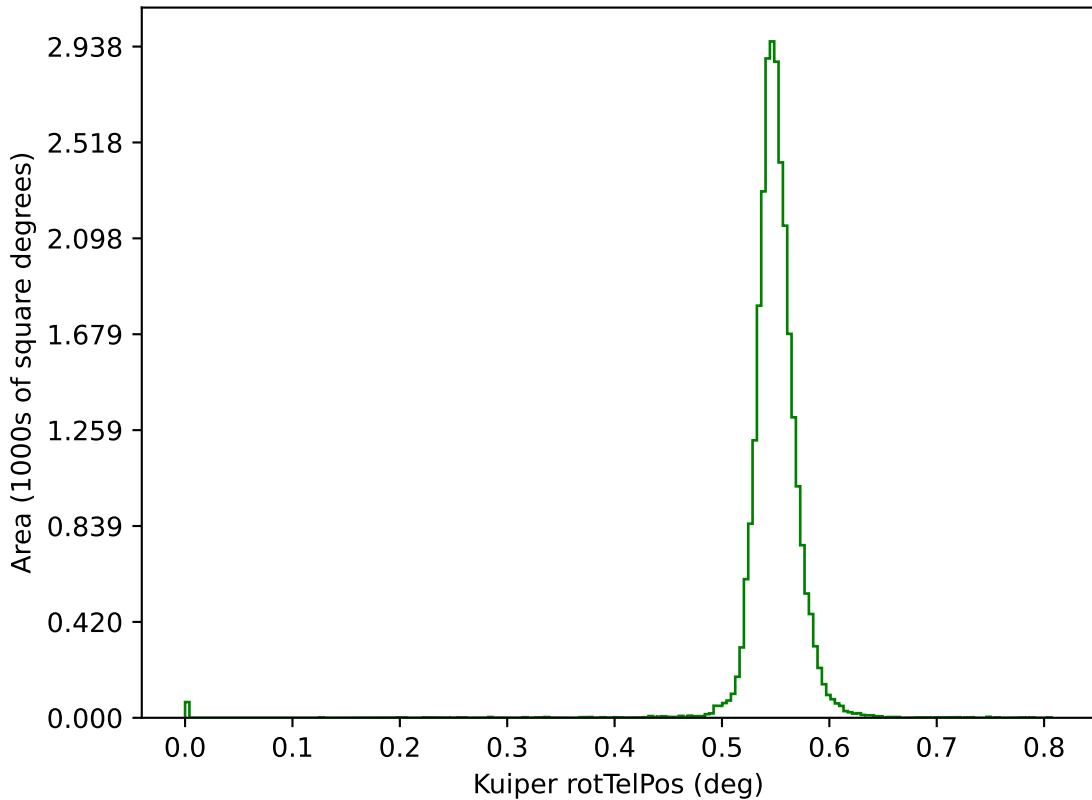
start_date_do-180v3.4_10yrs g: Kuiper rotTelPos
