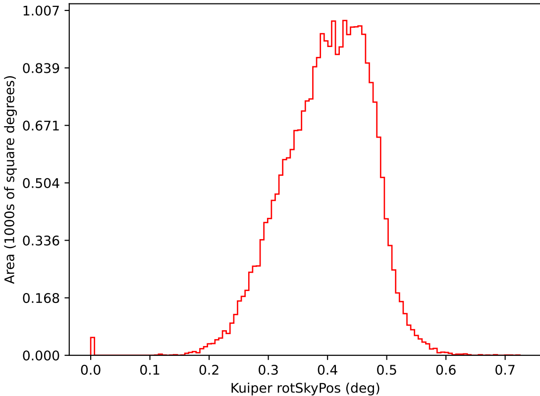
start_date_do-180v3.4_10yrs i: Kuiper rotSkyPos
