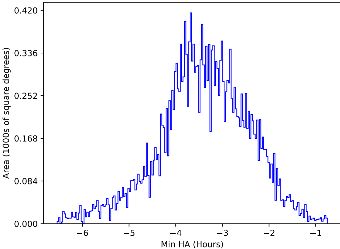
start_date_do-180v3.4_10yrs All sky y band: Min HA
