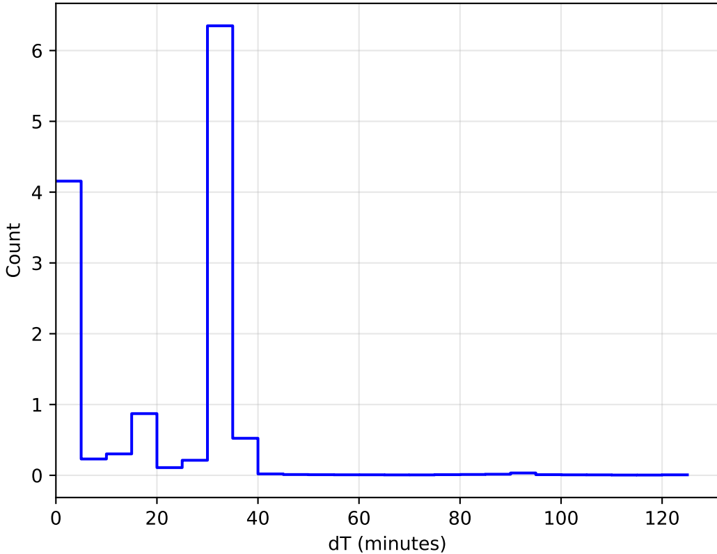
start_date_do-180v3.4_10yrs All sky: DeltaT Histogram
