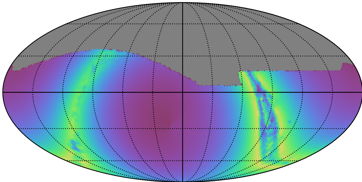
smc_lmc_v3.3_10yrs : young_stars
