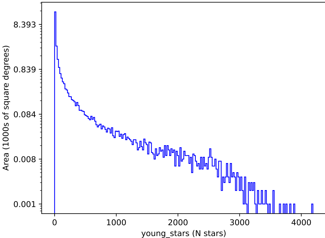
smc_lmc_v3.3_10yrs : young_stars
