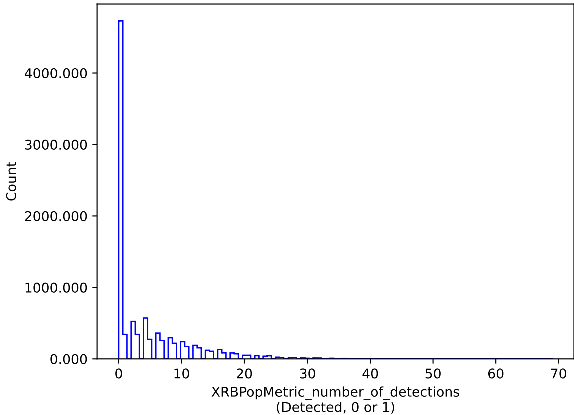
smc_lmc_v3.3_10yrs : XRBPopMetric_number_of_detections
