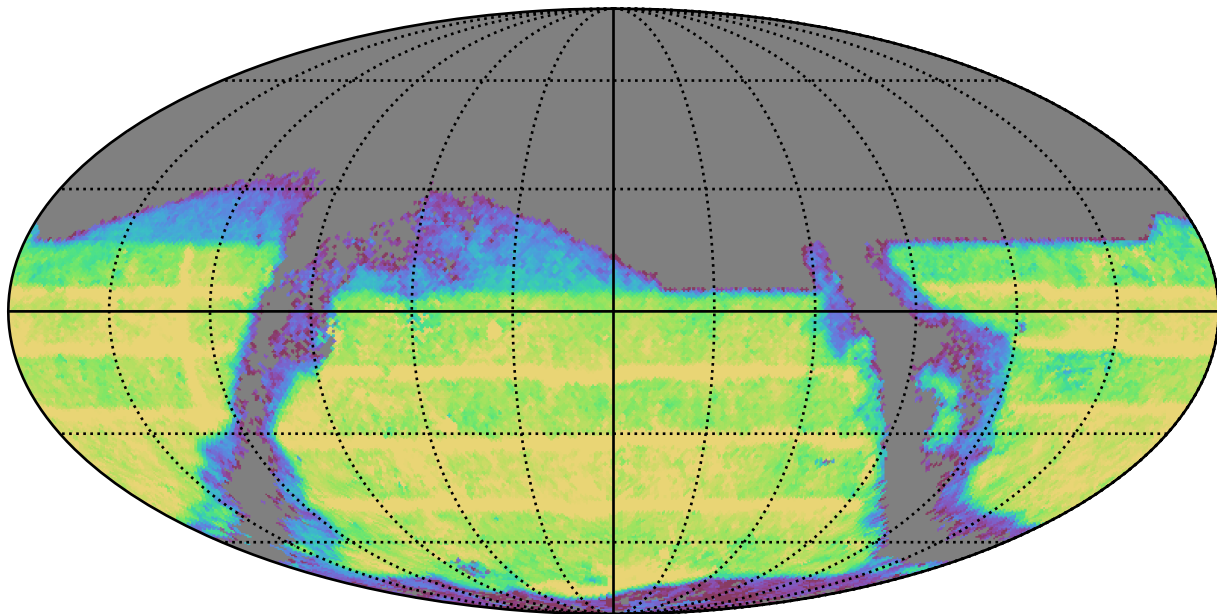
smc_lmc_v3.3_10yrs : TDC_rate
