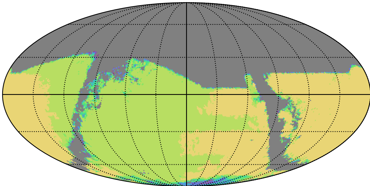
smc_lmc_v3.3_10yrs : TDC_campaign
