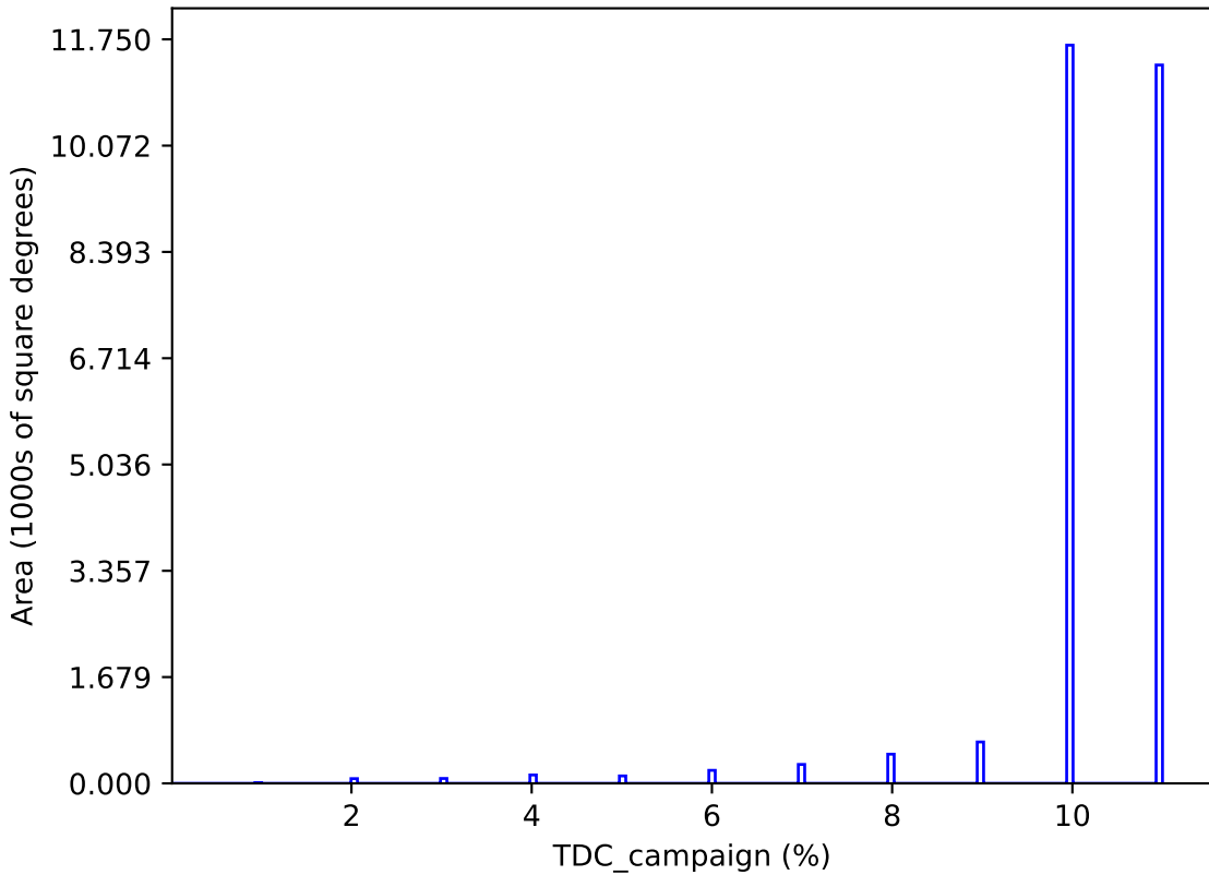
smc_lmc_v3.3_10yrs : TDC_campaign
