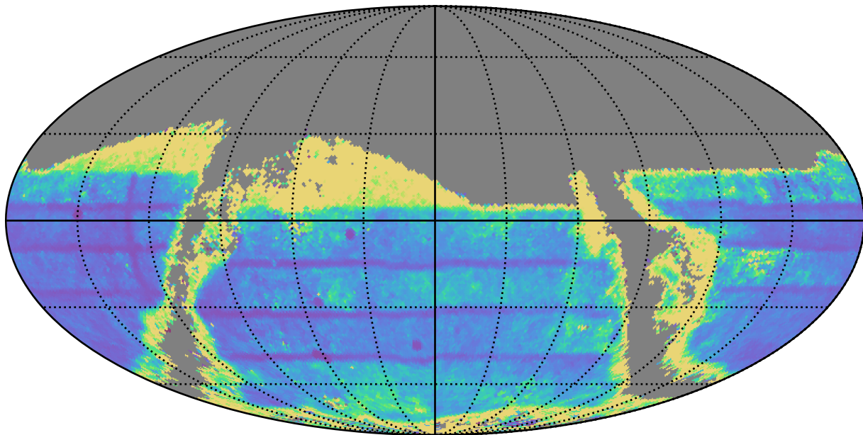
smc_lmc_v3.3_10yrs : TDC_cadence
