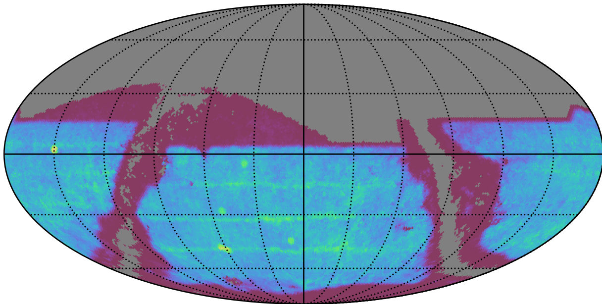
smc_lmc_v3.3_10yrs : SNSLMetric
