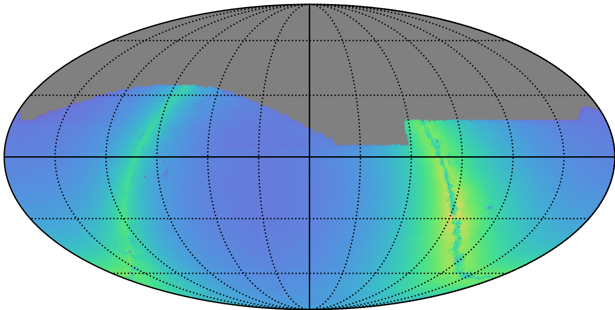
smc_lmc_v3.3_10yrs z: Nstars_no_crowding
