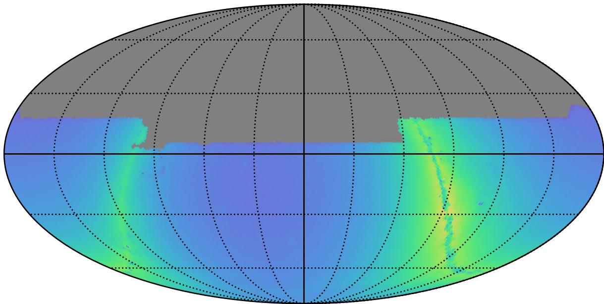
smc_lmc_v3.3_10yrs y: Nstars_no_crowding
