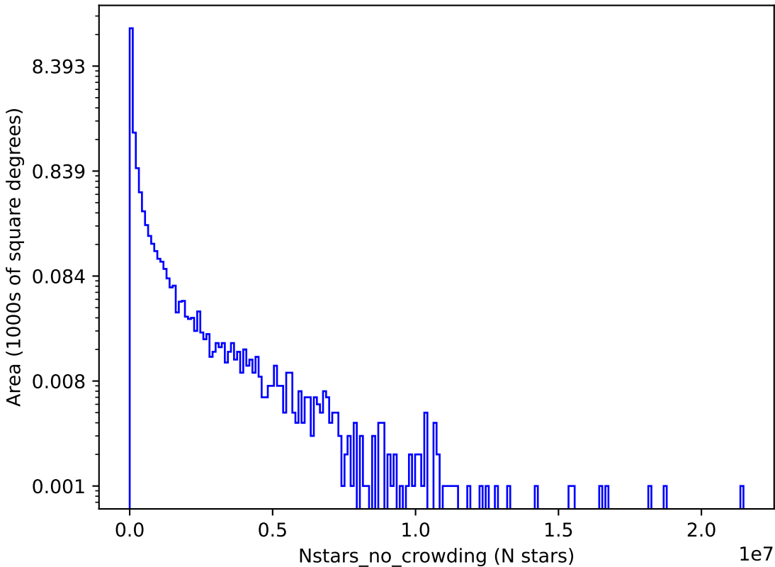
smc_lmc_v3.3_10yrs y: Nstars_no_crowding
