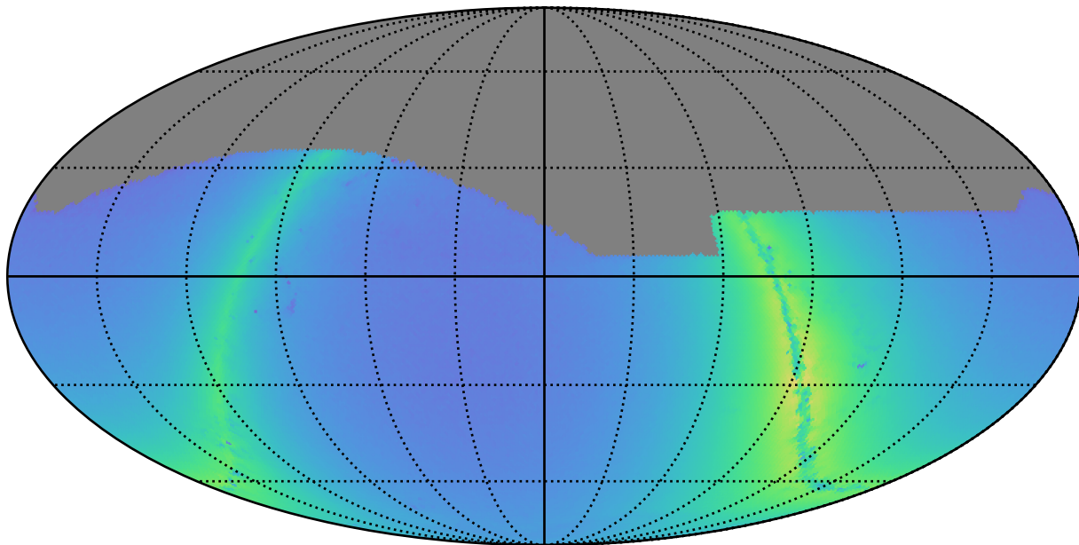
smc_lmc_v3.3_10yrs i: Nstars_no_crowding
