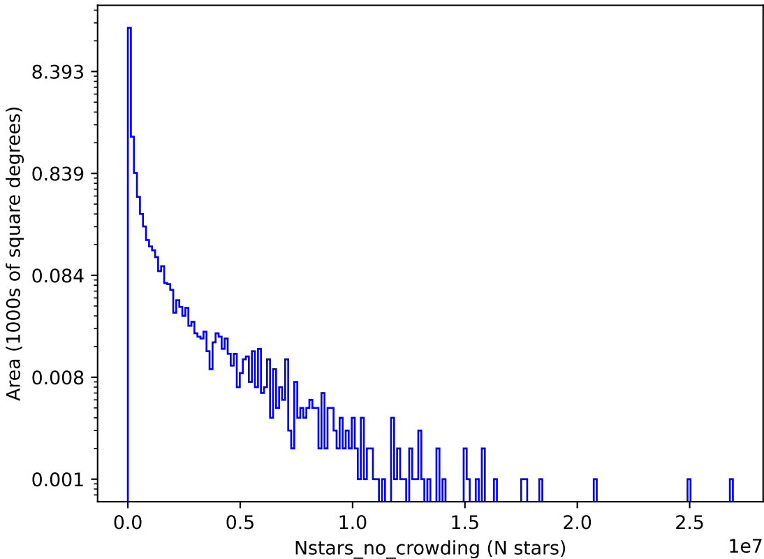
smc_lmc_v3.3_10yrs i: Nstars_no_crowding
