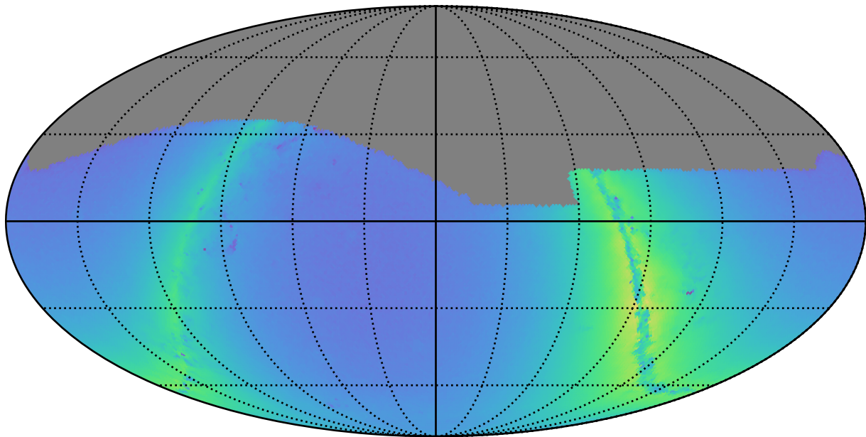
smc_lmc_v3.3_10yrs g: Nstars_no_crowding
