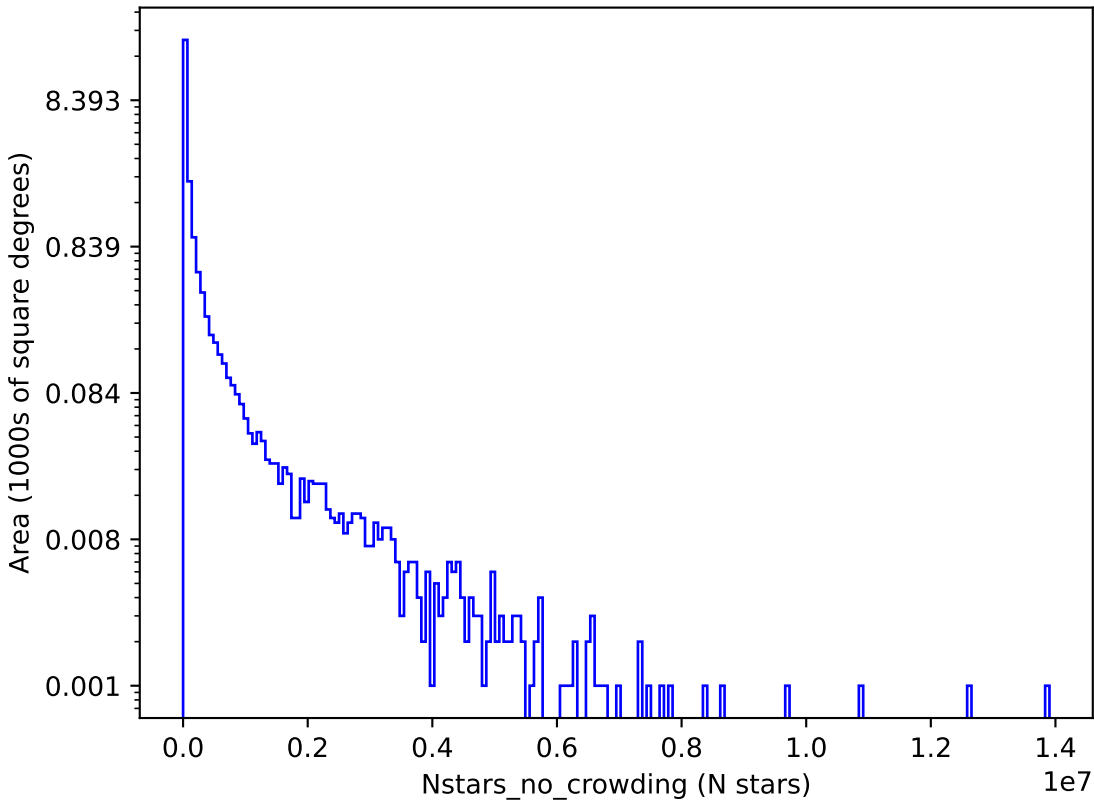
smc_lmc_v3.3_10yrs g: Nstars_no_crowding
