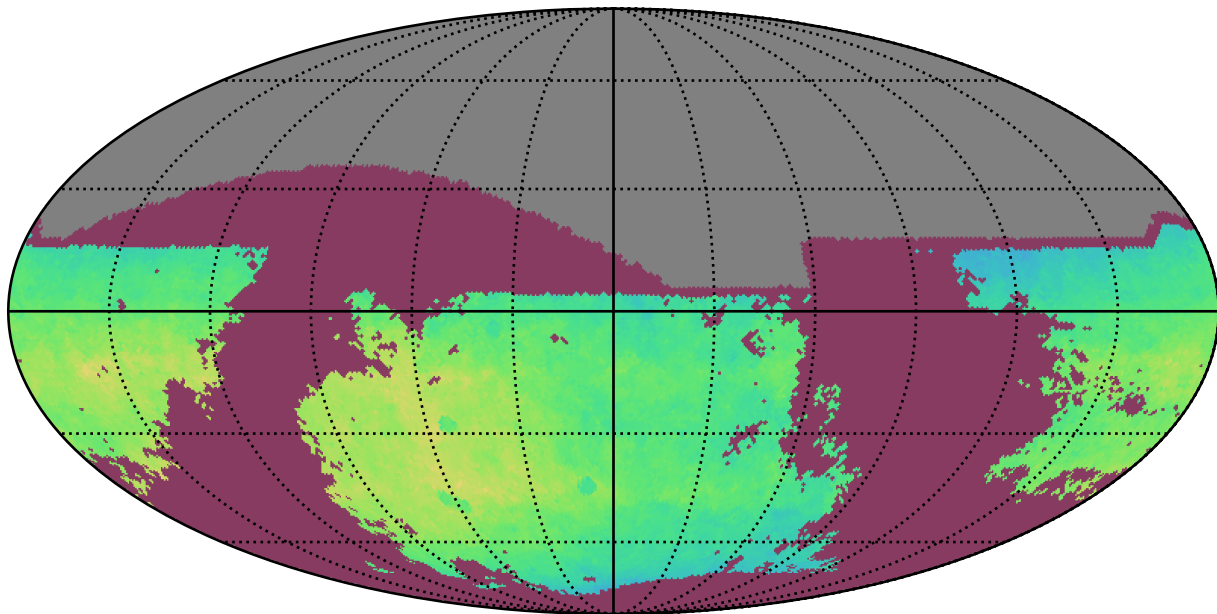
smc_lmc_v3.3_10yrs i: NgalScale
