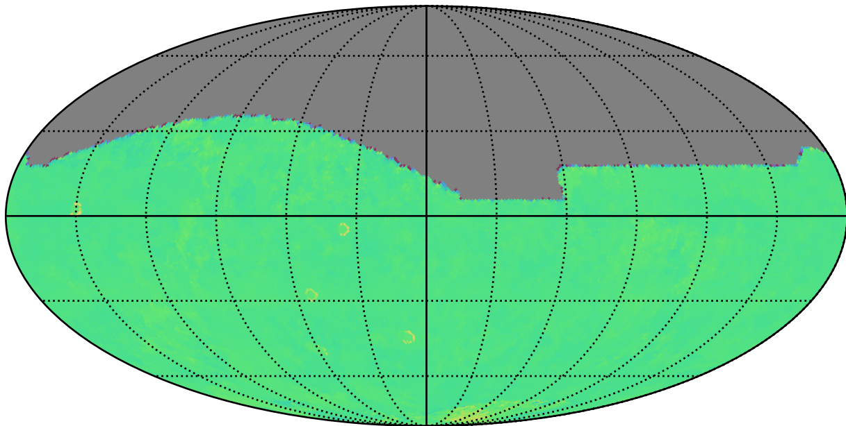
smc_lmc_v3.3_10yrs z: Kuiper rotTelPos
