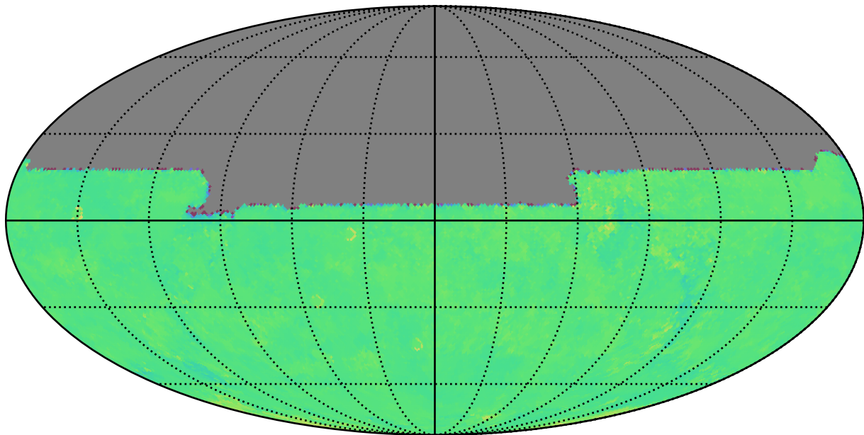
smc_lmc_v3.3_10yrs u: Kuiper rotTelPos
