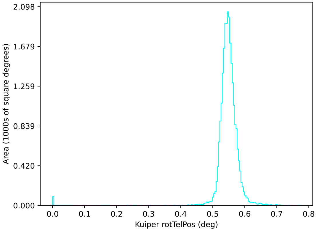
smc_lmc_v3.3_10yrs u: Kuiper rotTelPos
