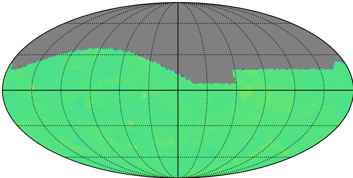
smc_lmc_v3.3_10yrs r: Kuiper rotTelPos
