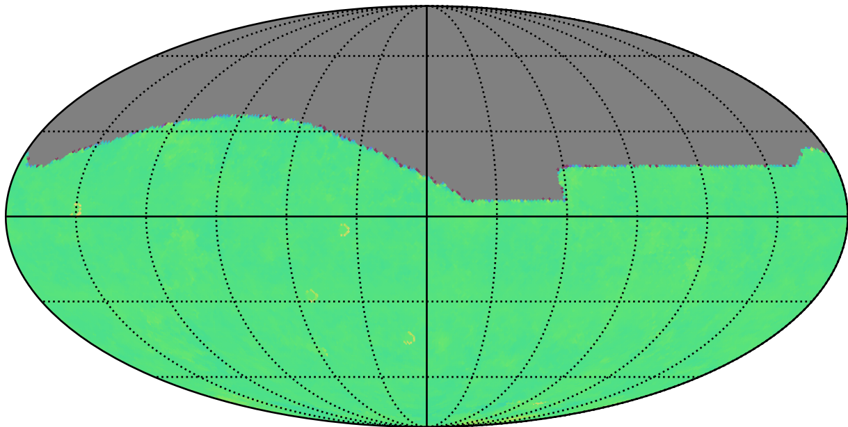
smc_lmc_v3.3_10yrs i: Kuiper rotTelPos
