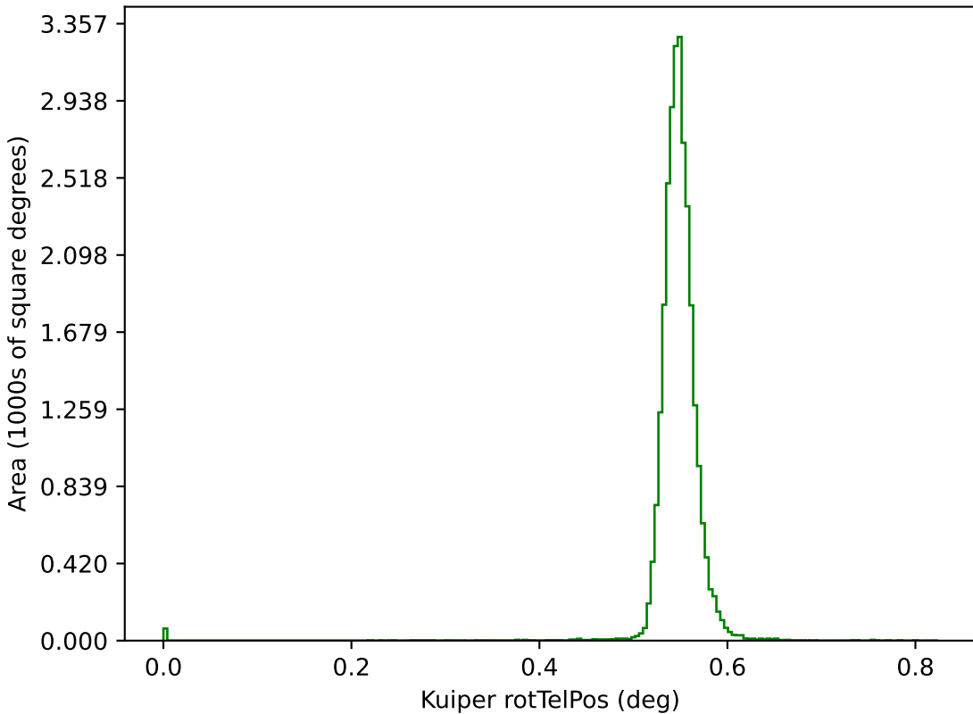
smc_lmc_v3.3_10yrs g: Kuiper rotTelPos
