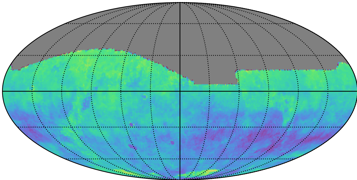
smc_lmc_v3.3_10yrs z: Kuiper rotSkyPos
