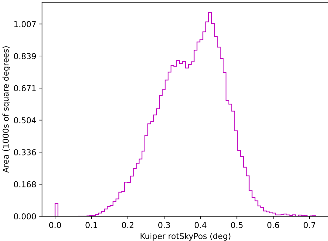
smc_lmc_v3.3_10yrs z: Kuiper rotSkyPos
