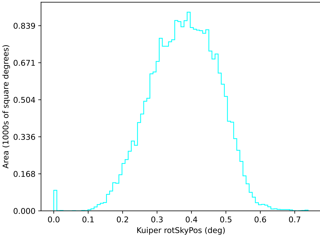
smc_lmc_v3.3_10yrs u: Kuiper rotSkyPos
