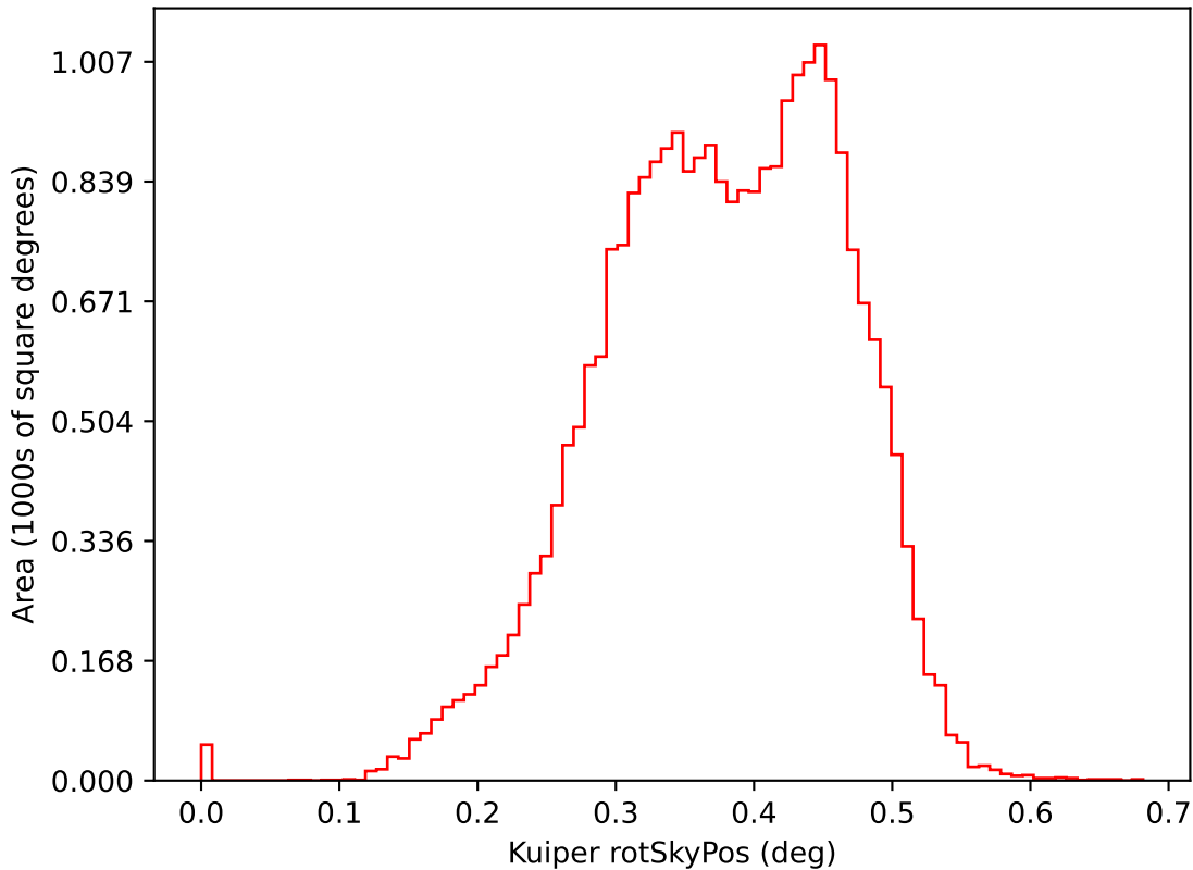
smc_lmc_v3.3_10yrs i: Kuiper rotSkyPos
