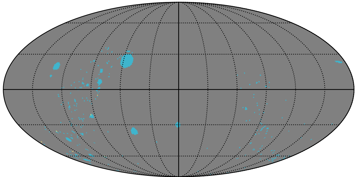
smc_lmc_v3.3_10yrs : GalplaneFootprintMetric_open_clusters_map_Tau_5_0
