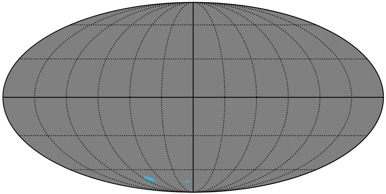
smc_lmc_v3.3_10yrs : GalplaneFootprintMetric_magellanic_clouds_map_Tau_46_5
