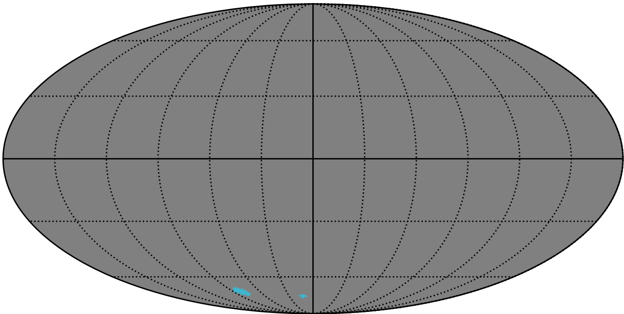
smc_lmc_v3.3_10yrs : GalplaneFootprintMetric_magellanic_clouds_map_Tau_2_0
