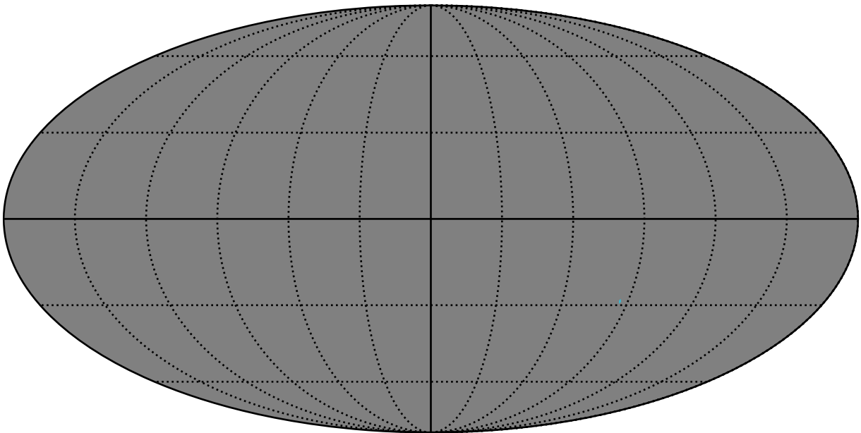
smc_lmc_v3.3_10yrs : GalplaneFootprintMetric_globular_clusters_map_Tau_46_5
